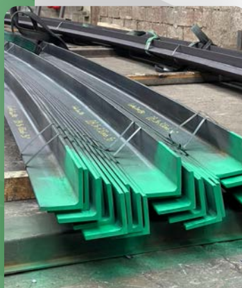
cornières 120x80x10 avec échancrures
